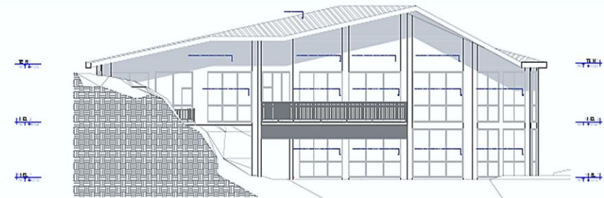
ELEVACION FRONTAL ESCALA 1/75
