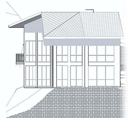
ELEVACION LATERAL
